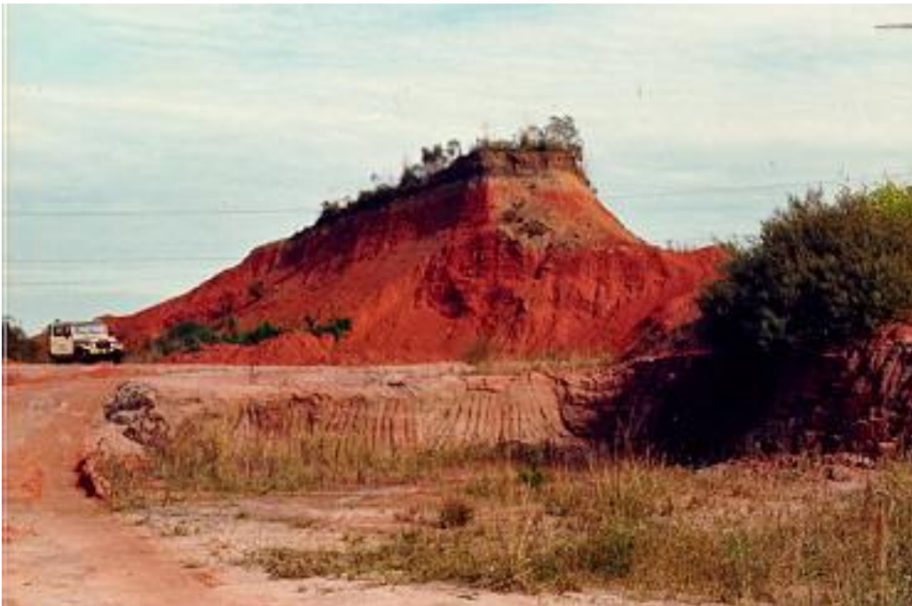
Figura 6. Afloramento do SAG Triássico representado pela Formação Santa Maria (Membros Alemoasíltico-argiloso avermelhado e Passo das Tropas arenoso rosado) no Compartimento Central.
