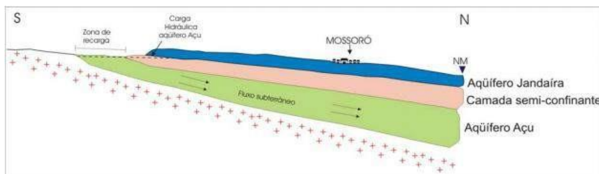
Figura 4: Seção esquemática das unidades Hidrogeológicas da Bacia Potiguar.
