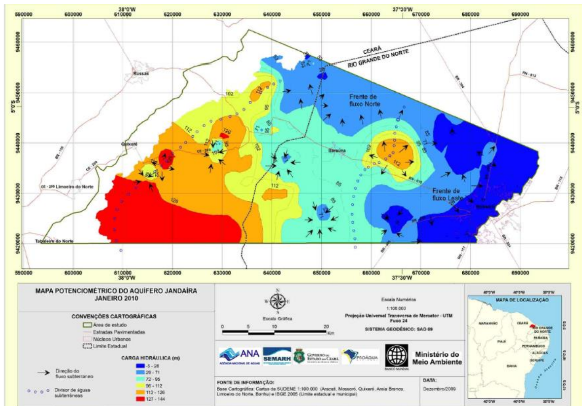
Figura 5 – Potencimetria do Aquífero Jandaíra em Janeiro de 2010. Fonte: ANA, 2010.
