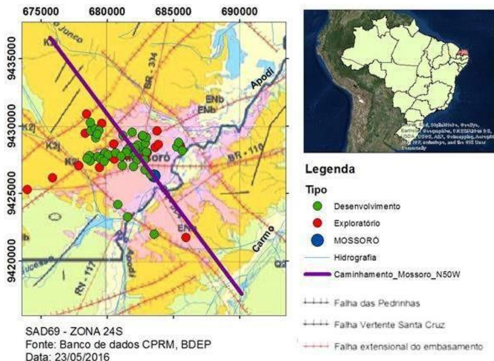
Figura 8: Mapa geológico referenciando as principais falhas da região em estudo. Fonte: Adaptado do ProÁgua (2010).
