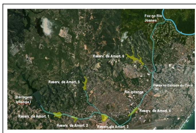
Figura 3. Localização dos Reservatórios de Amortecimento propostas
