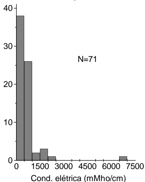
Gráfico 13. Frequência de Condutividade Elétrica no Grupo Macaúbas
