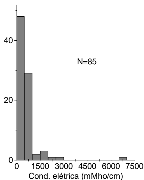
Gráfico 14. Frequência de Condutividade Elétrica na área
