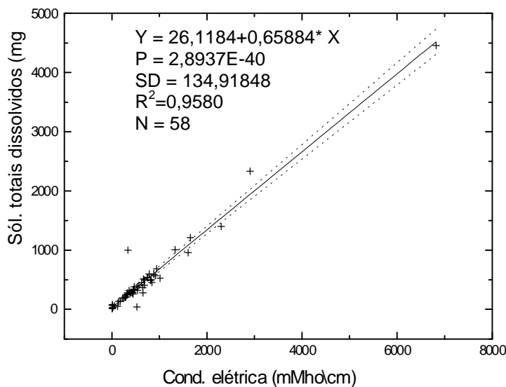
Gráfico 15. Correlação entre condutividade elétrica e sólidos totais dissolvidos na área.
