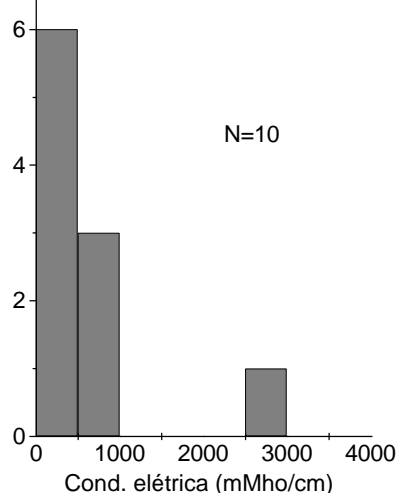
Gráfico 12. Frequência de Condutividade Elétrica nos granitóides
