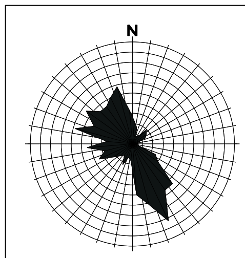
Figura 04. Diagrama em rosácea de juntas na área. N=400
