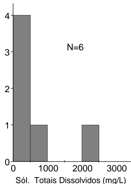
Gráfico 08. Frequência de STD nos granitóides
