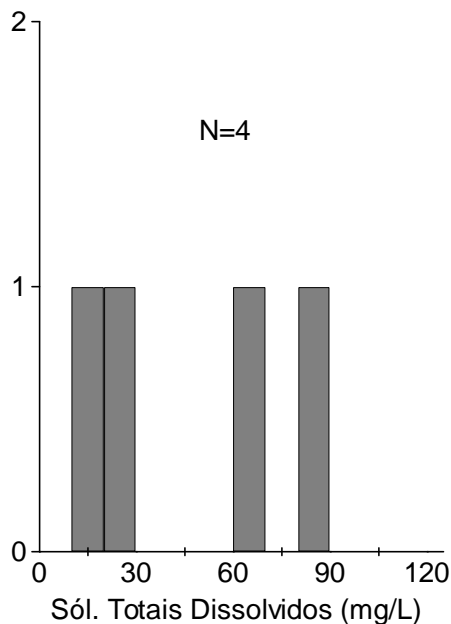
Gráfico 07. Frequência de STD na Fm. São Domingos
