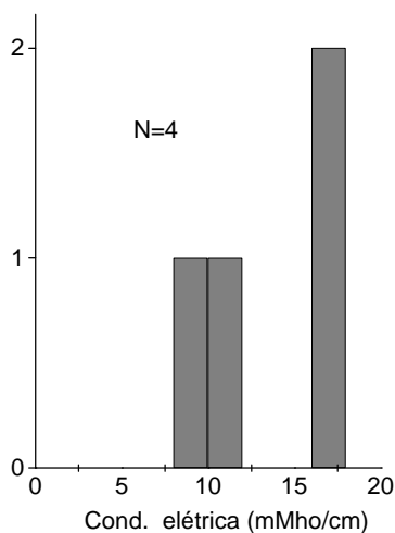
Gráfico 11. Frequência de Condutividade Elétrica na Fm. São Domingos
