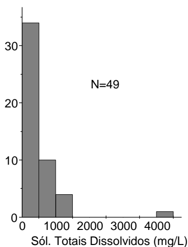
Gráfico 09. Frequência de STD no Grupo Macaúbas
