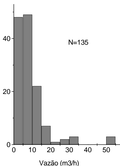
Gráfico 03. Frequência de vazão no Grupo Macaúbas
