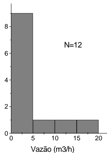
Gráfico 02. Frequência de vazão nos granitóides
