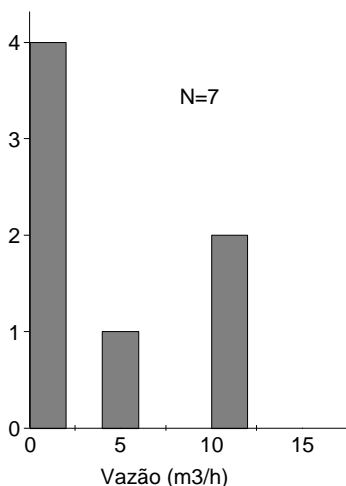
Gráfico 01. Frequência de vazão na Fm. São Domingo
