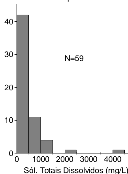
Gráfico 10. Frequência de STD na área
