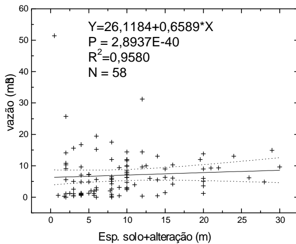
Gráfico 05. Correlação entre espessura do solo + alteração e vazão na área
