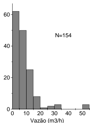
Gráfico 04. Frequência de vazão na área total
