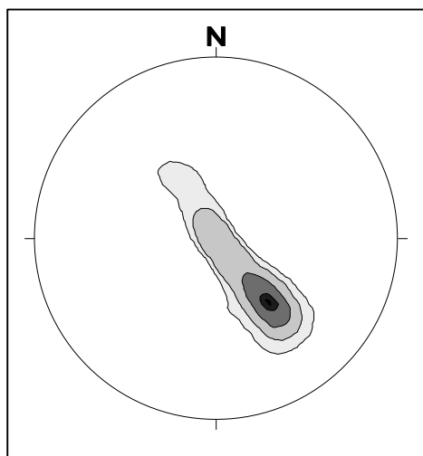
Figura 03. Isolinhas de RMD da xistosidade do Grupo Macaúbas. conc. máx. 141^{\circ}/53^{\circ} 2,07%-6,21%-16,21%-25,17%-27,93% N=290
