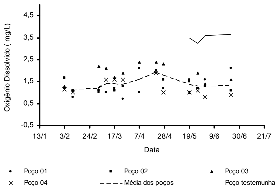
Figura 4 - Variação temporal da concentração de Oxigênio Dissolvido nos poços de observação localizados junto às faixas de tratamento de esgoto por escoamento superficial.
