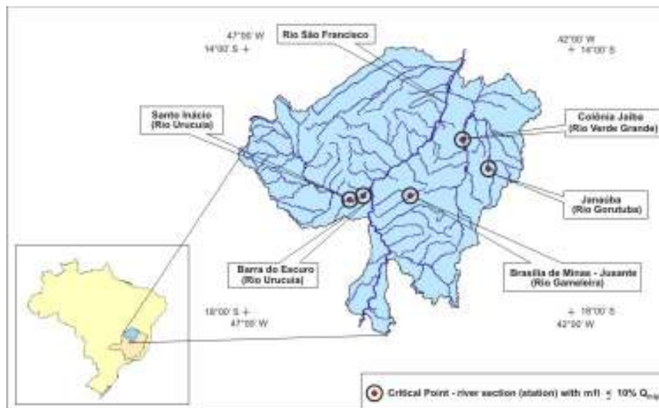
Figura 2. Localizações das seções fluviais que apresentaram baixa capacidade de regularização natural, na região hidrográfica do Alto Médio São Francisco, em Minas Gerais.
