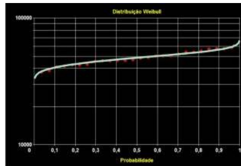
Figura 2. Ajuste da distribuição de Weibull às vazões mínimas do rio Carinhanha em São Gonçalo.
