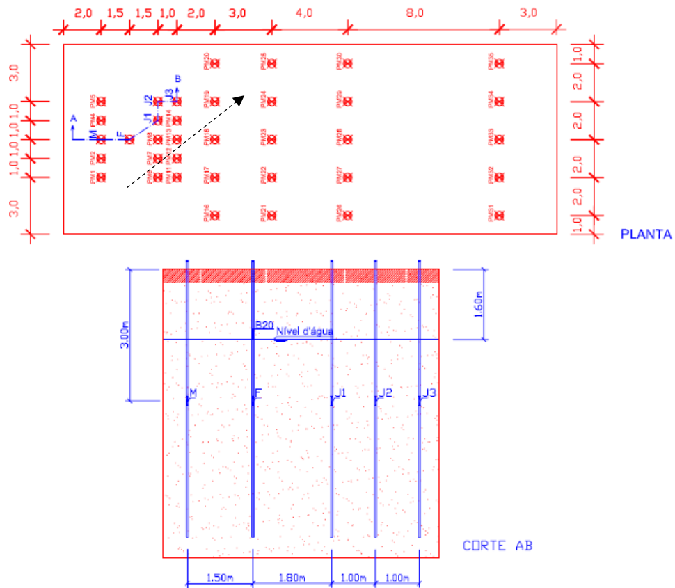
Figura 1: Planta e corte da área B20 (80% de diesel e 20% de biodiesel). Poços analisados: Fonte (F), poços a jusante (J) de F (J1 a 1,5m de F; J2 a 2,5m de F; e J3 a 3,5m de F) e um poço a montante de F (M a 1,5m de F). A profundidade da amostragem foi de 3m em relação á cota do terreno. Comportamento horizontal.
