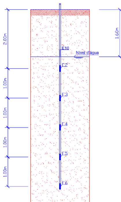
Figura 2: Área E10, a amostragem foi realizada na fonte, poço onde foi liberado o combustível E10, nas diferentes profundidades, 2m (F2), 3m (F3), 4m (F4), 5m (F5) e 6m (F6) em relação à cota do terreno. Comportamento vertical.
