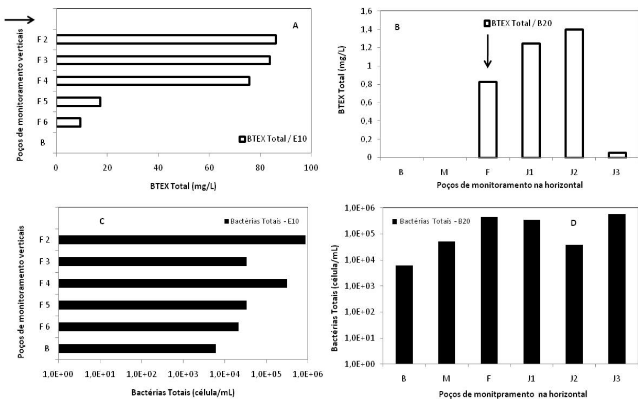
Figura 3: Concentração dos compostos BTEX da área E10 (A) e da área B20 (B); bactérias totais da área E10 (C) e da área B20 (D). As setas indicam o ponto onde foi liberado os contaminantes. Os dois gráficos da esquerda mostram a área em que foi feita a análise vertical com amostras de diferentes profundidades na fonte F (F2 a 0,5m do nível da água, F3 a 1,5m, F4 a 2,5m; F5 a 3,5m e F6 a 4,5m do nível da água). Os gráficos á direita mostram poços a jusante (J) da fonte F (J1 a 1,5m de F; J2 a 2,5m de F; e J3 a 3,5m de F) e um poço a montante (M a 1,5m de F). A letra B (branco) indica o ponto controle dos experimentos.
